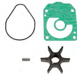
18-3285 KIT SERVICIO BOMBA DE AGUA Reemplaza: 06192-ZY3-000 Para: BF200/225 Incluye impulsor 18-3031
