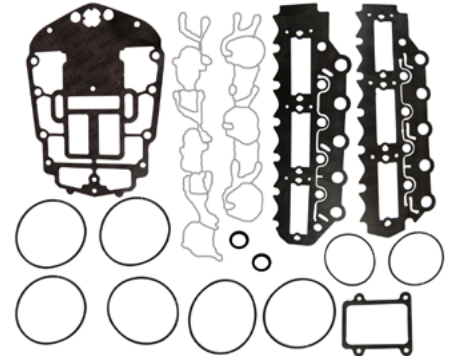
18-4406 KIT JUNTAS MOTOR Reemplaza: 437155 Para: 150 60 grados (1991-00), 175 60 grados (1991-00)
