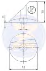
025741 Zn 0,33 Tohatsu. Ánodo aleta para estabilizador motor fueraborda Tohatsu 2T 25-50HP, 4T 25-30HP. #OEM 387-60217-0
