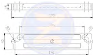
025742 Zn 0,5 Tohatsu Barra para transom fueraborda Tohatsu 2T 40-140 HP. #OEM 3C7-60218-2
