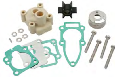
18-48317 KIT BOMBA DE AGUA COMPLETO Reemplaza: 3B2-87322-0 Para: F8/9.8
