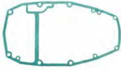
18-99013 JUNTA CÁRTER SUPERIOR Reemplaza: 66M-45113-00 Para: F9.9 (2005-06), F15(1998-05), T9.9(2005-06)
