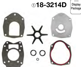
18-3214 KIT BOMBA AGUA Reemplaza: 19021-ZW1-003 Para: BF 70/BF 90 1996-98 Incluye impulsor 18-3056
