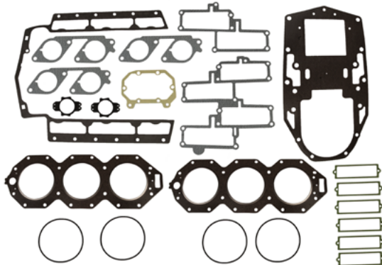
18-4428 KIT JUNTAS MOTOR Reemplaza: 437725 Para: 200 BB (1993 & sup), 225 BB (1993 & sup), 225 Ficht FFI (1999 & sup), 250 solo Carb (2000)
