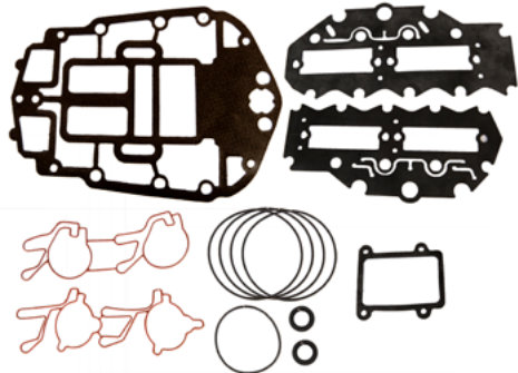
18-4402 KIT JUNTAS MOTOR Reemplaza: 437779, 439559 Para: 90 V4 60 grados (1995-00), 115 V4 60 grados (1995-00)
