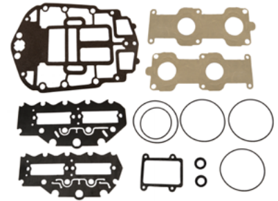
18-4406 KIT JUNTAS MOTOR Reemplaza: 437155 Para: 150 60 grados (1991-00), 175 60 grados (1991-00)
