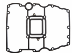
18-99028 JUNTA CÁRTER Reemplaza: 68V-15312-00 Para: F75(2003-10), F90(2004-10), F115(2004-10), LF115(2004-10)
