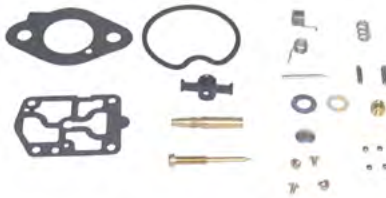
18-7226 KIT CARBURADOR Reemplaza: 1395-9650 Para: 30 JET, 40/45 4 Cil 4 Tiempos, Carb modelos WMA-7B,9,10,13
