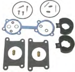
18-7290* KIT CARBURADOR Reemplaza: 696-W0093-02-00 *kit contiene componentes suficientes para reconstruir 2 carburadores
