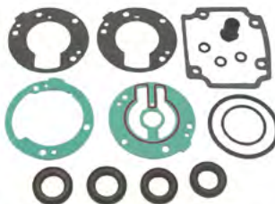
18-2785 KIT RETÉN ALOJAMIENTO ENGRANAJE Reemplaza: 689-W0001-21-00, 689-W0001-C1-00
