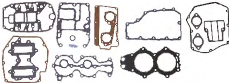
18-4305 KIT JUNTAS MOTOR Reemplaza: 393433, 437806, 439083 Para: sólo modelos 2 cilindros
