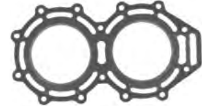
18-3822 JUNTA CULATA Reemplaza: 11141-87E90, 11141-87E10
