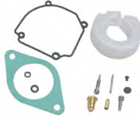
18-7291 KIT CARBURADOR Reemplaza: 6H1-W0093-01-00 (3) de 18-7291 = (1) de 6H1-W0093-01-00
