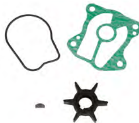
18-3281 KIT SERVICIO BOMBA DE AGUA Reemplaza: 06192-ZV7-000 Para: BF25/30 Incluye impulsor 18-3249
