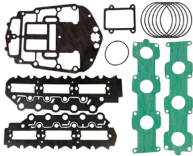
18-4402 KIT JUNTAS MOTOR Reemplaza: 437779, 439559 Para: 90 V4 60 grados (1995-00), 115 V4 60 grados (1995-00)
