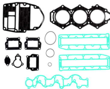
18-4435 JUEGO JUNTAS CULATA Reemplaza: 3F3-87121 Para: Todos 60-70 HP
