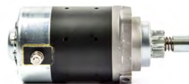
18-6418 MOTOR ARRANQUE Reemplaza: Tohatsu 353-76010-4 Para: M45A2, M50C, M60A, M70A2, M90A, M140A, NS45A2, NS50C, NS60A, NS70A2, NS90A, NSD90A, NS120A, NS140A (9 dientes)
